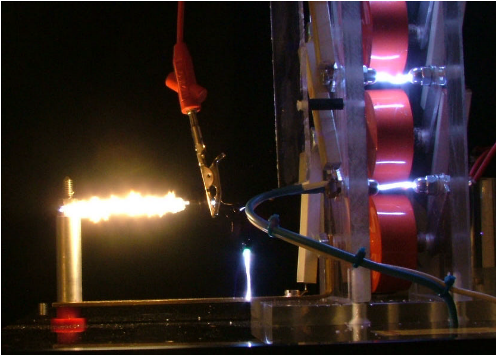
Drahtexplosion mittels Marxgenerator
