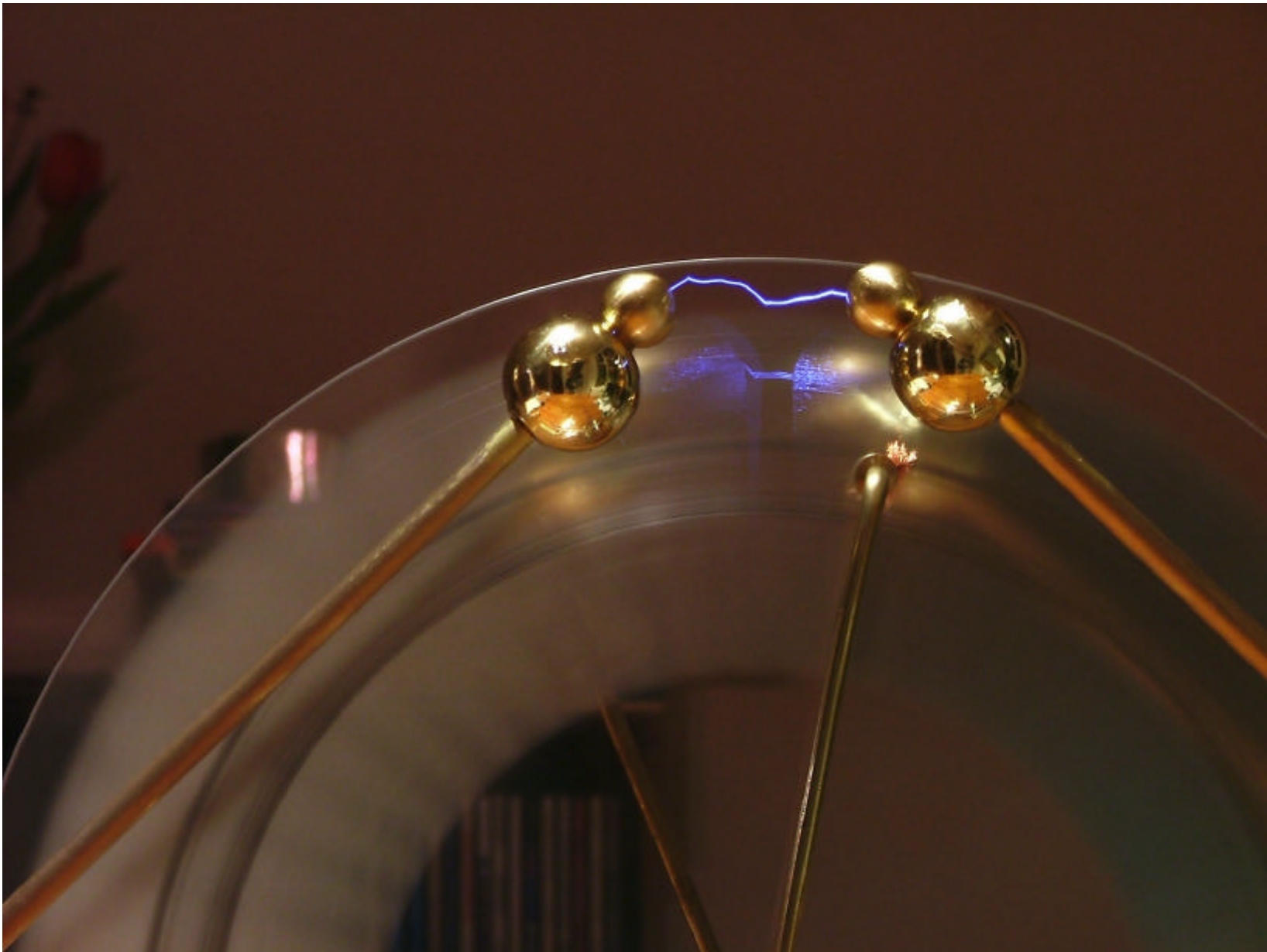
Funken an einer Influenzmaschine
