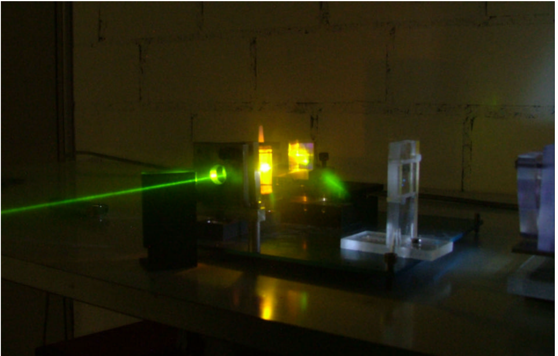
Strahl eines Rhodamin 6G Lasers
