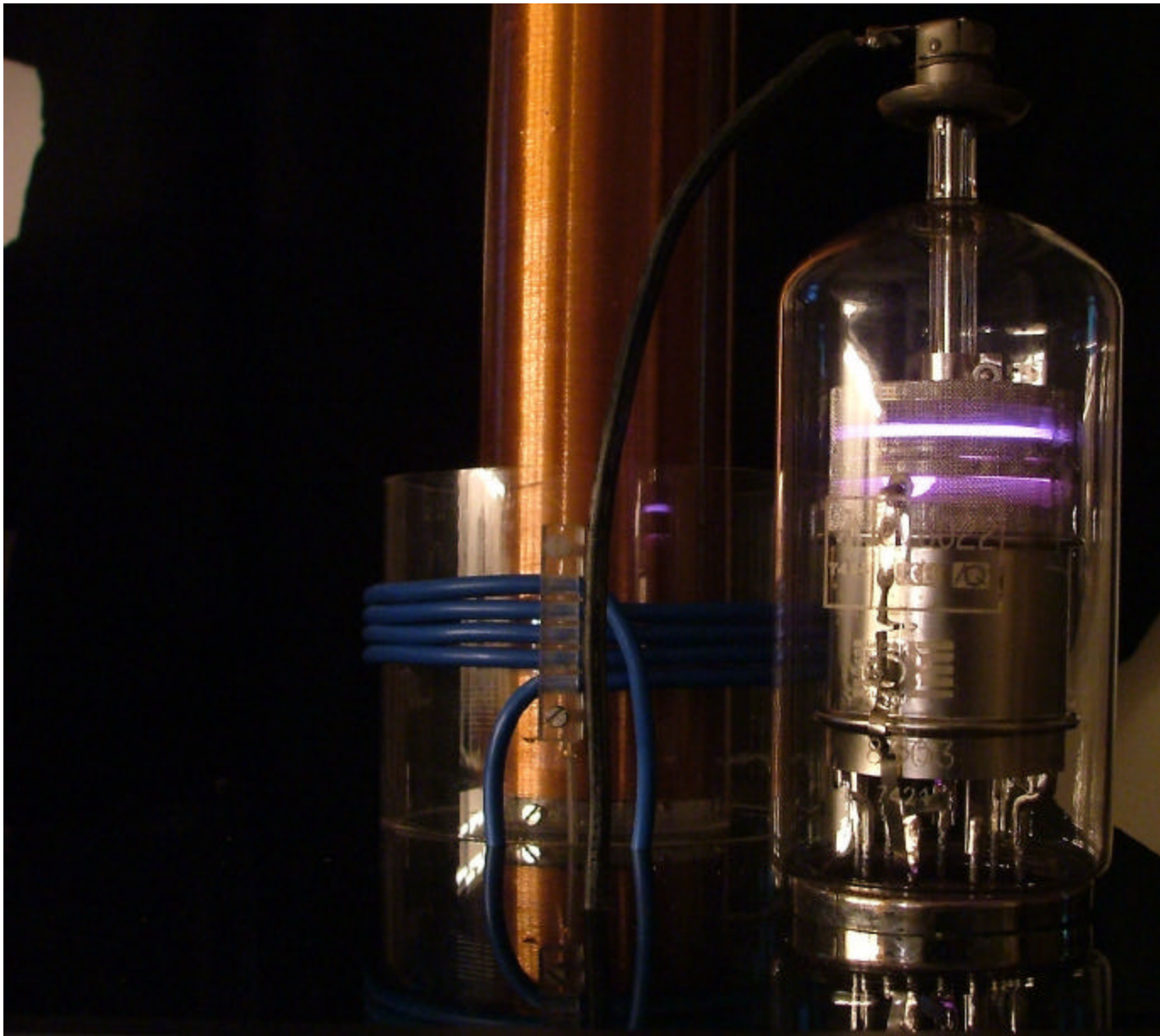
Betrieb eines Wasserstoff Thyratrons
