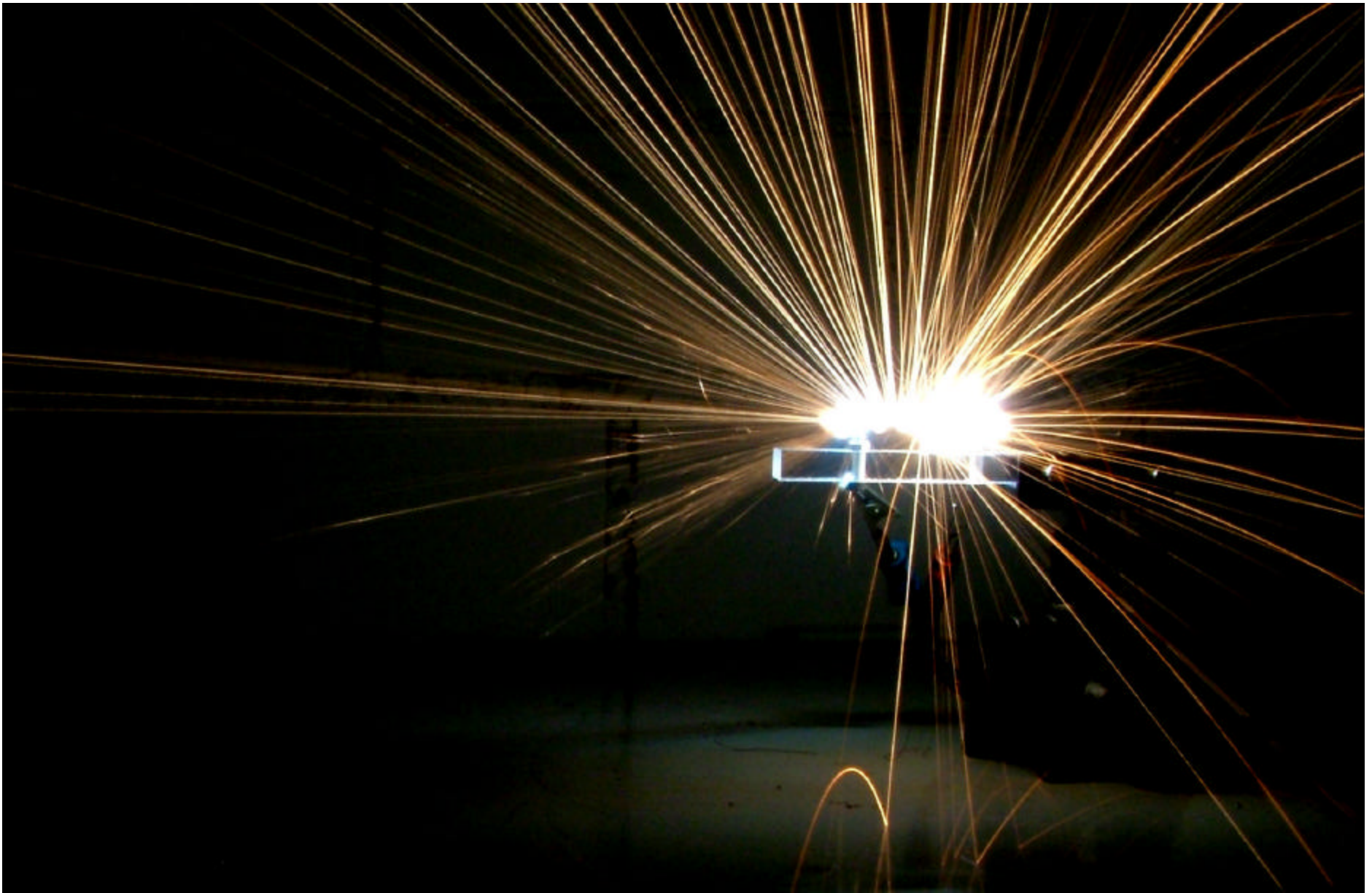
Drahtexplosion durch Kondensatorentladung
