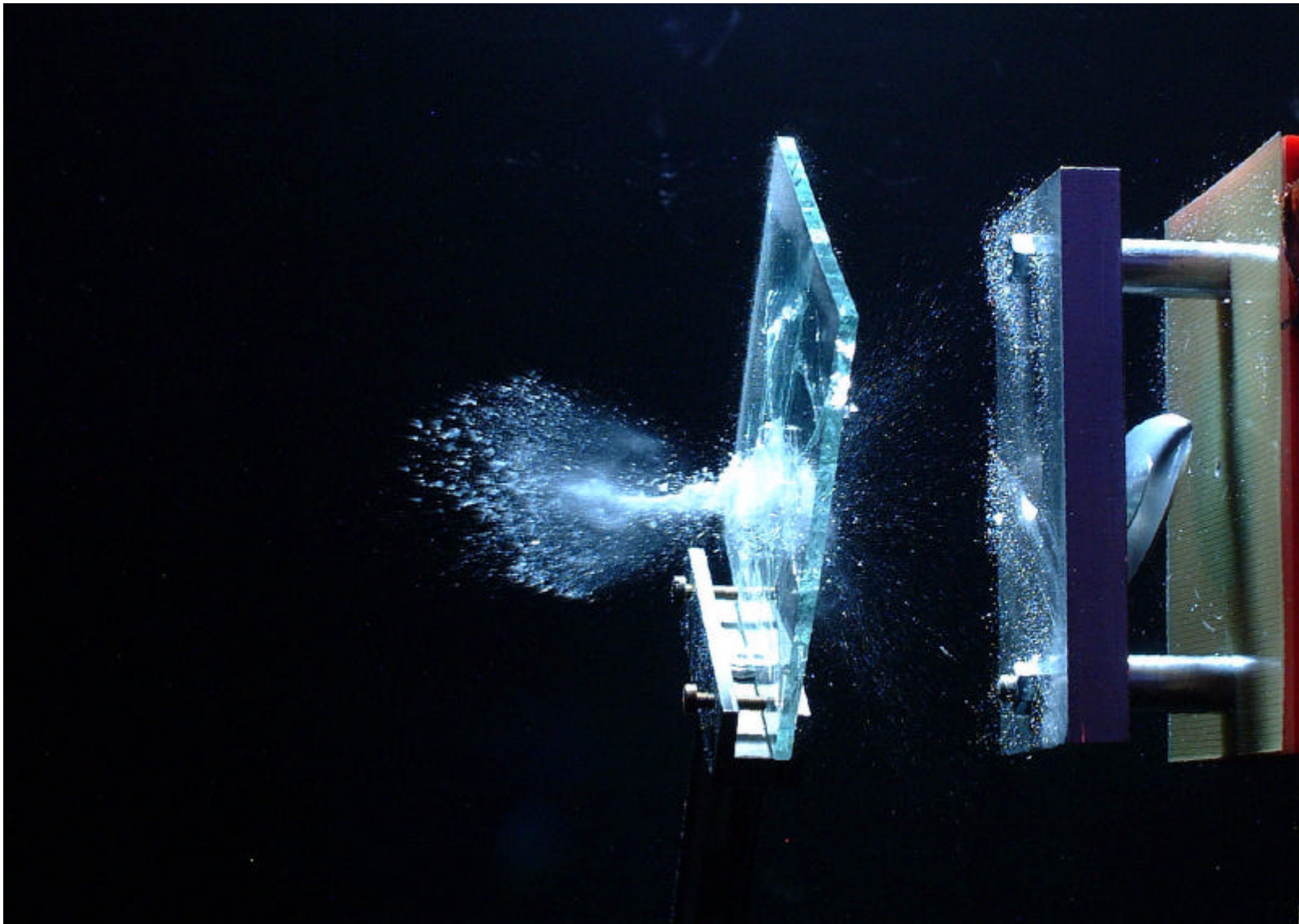
Eine mittels Wirbelstrom auf 830 kmh beschleunigte Stahlkugel zerstört eine Glasplatte
