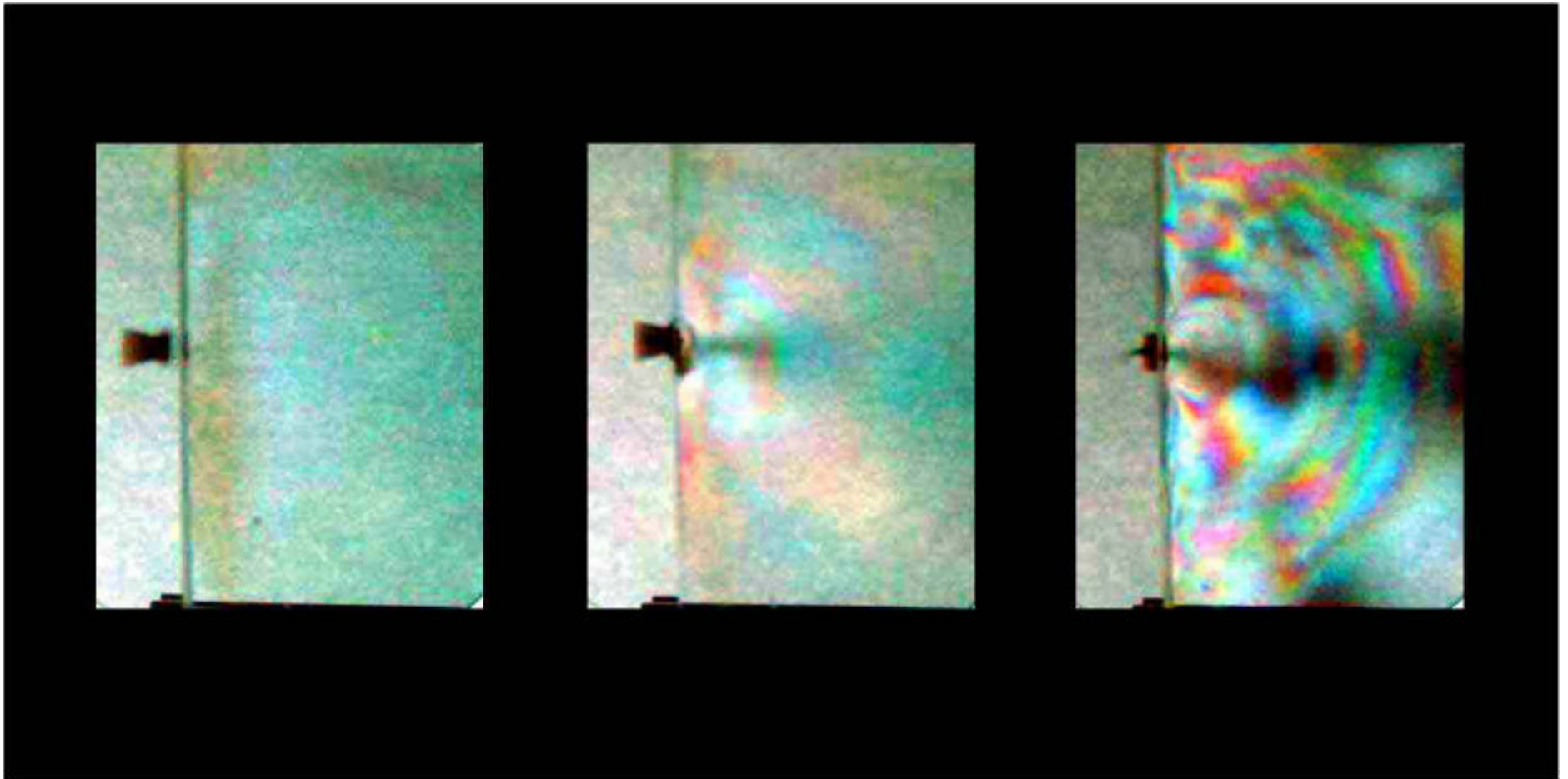
Schockwellen in einem Plexiglasblock, durch ein Luftgewehrgeschosses ausgelöst
